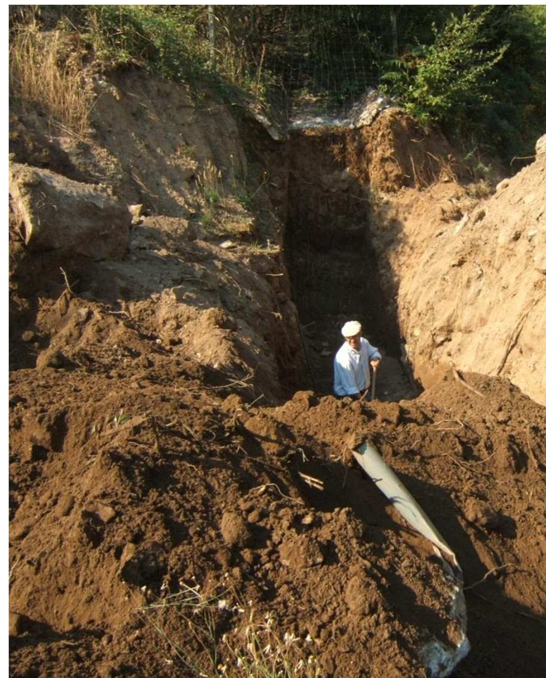
Execução de rede de drenagem de águas pluviais no caminho entre os lugares de Bouça e Vilar, Faia
